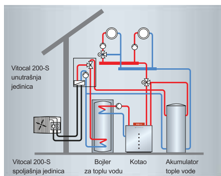
Šematski prikaz instalacije grejanja sa uređajem Vitocal 200-S za novogradnju (slika gore) i modernizaciju (slika dole)
